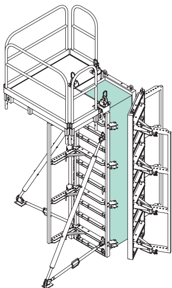
1. Napínací prvok uvoľniť a odklopiť prvý stĺpcový panel.
