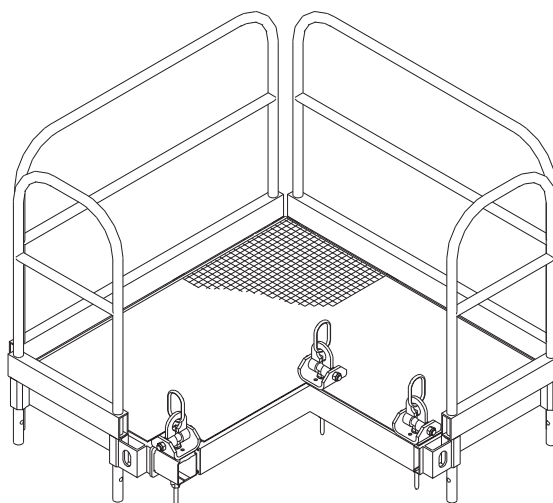
PERI betonárska plošina komplet, č. výr.: 037400
