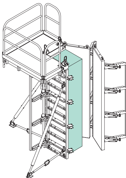
2. Potom uvoľnite od betónu druhý panel. Obidva panely zaistiť čapmi v otvorenej polohe (pozri detail).
